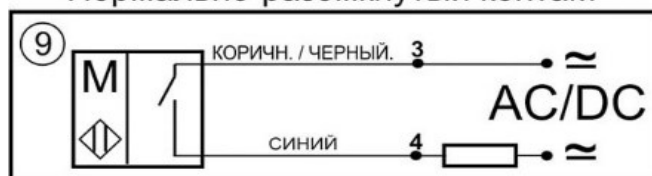
Схема соединения
