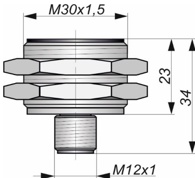
Габаритный чертеж
