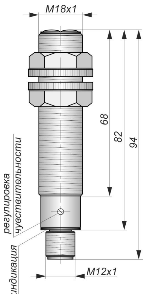
Габаритный чертеж
