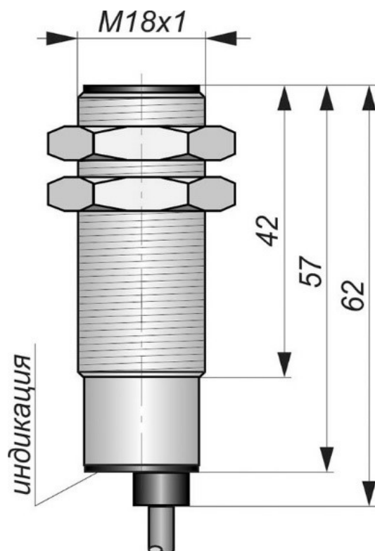
Габаритный чертеж
