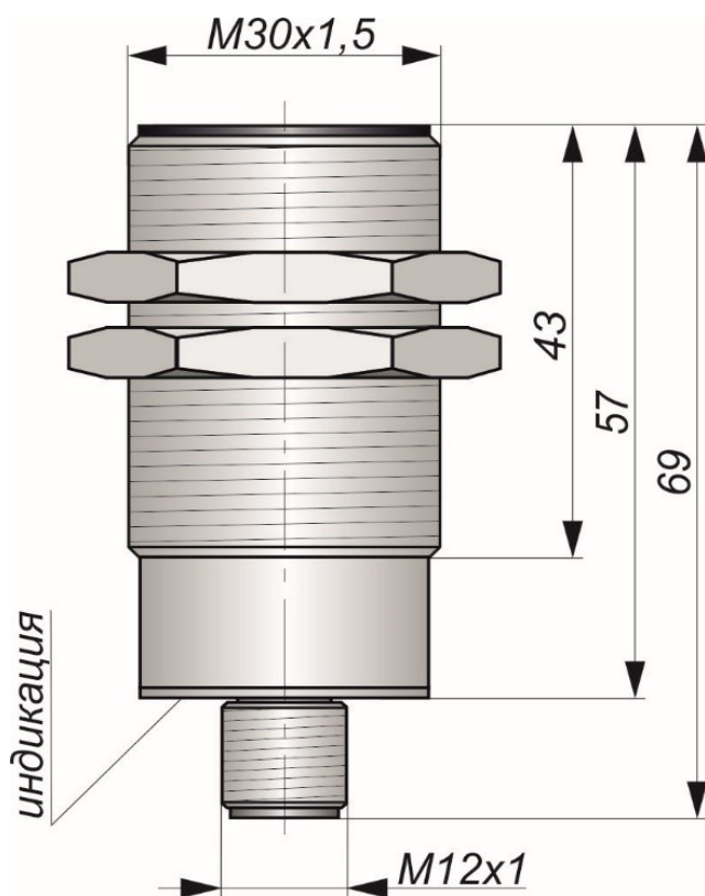
Габаритный чертеж
