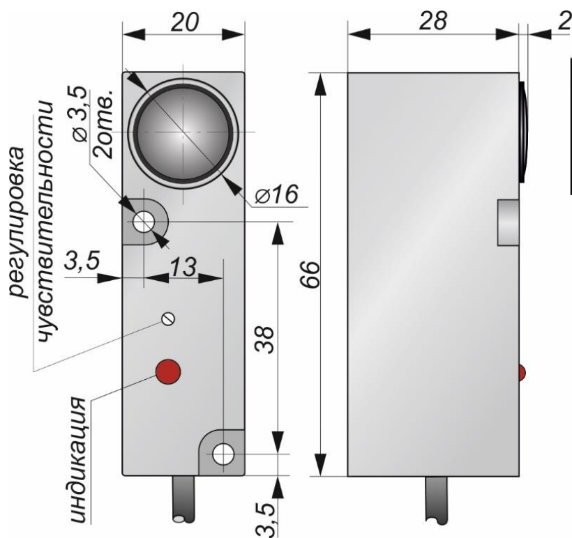
Габаритный чертеж
