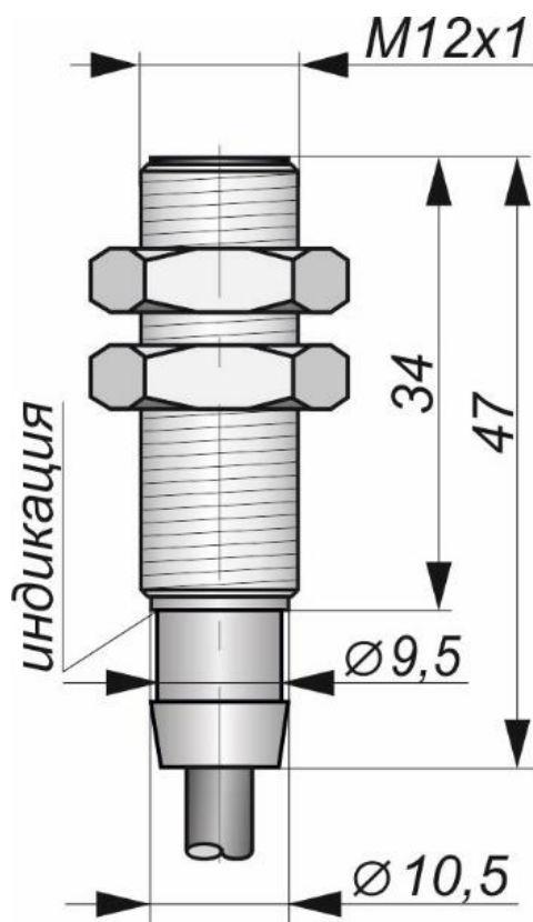
Габаритный чертеж
