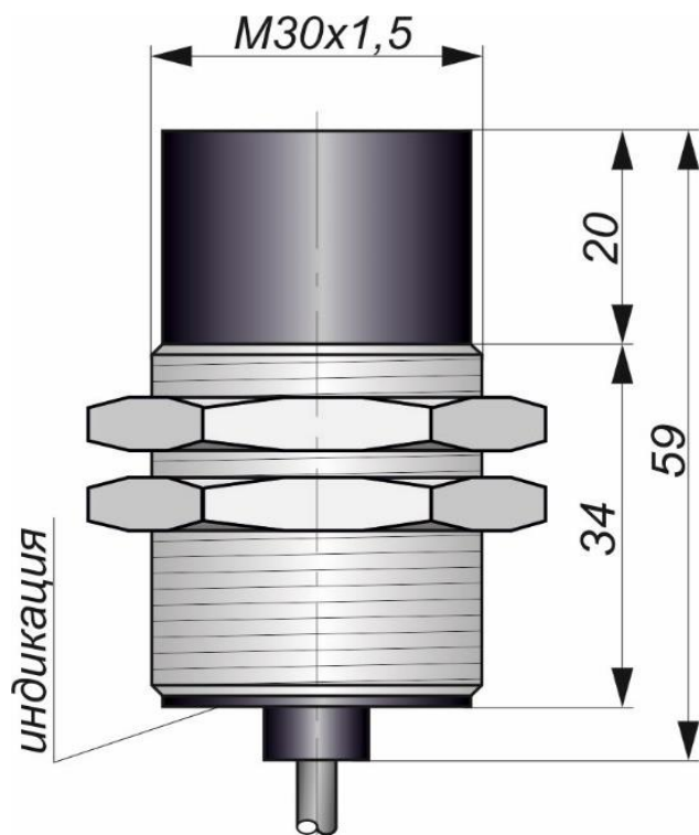
Габаритный чертеж
