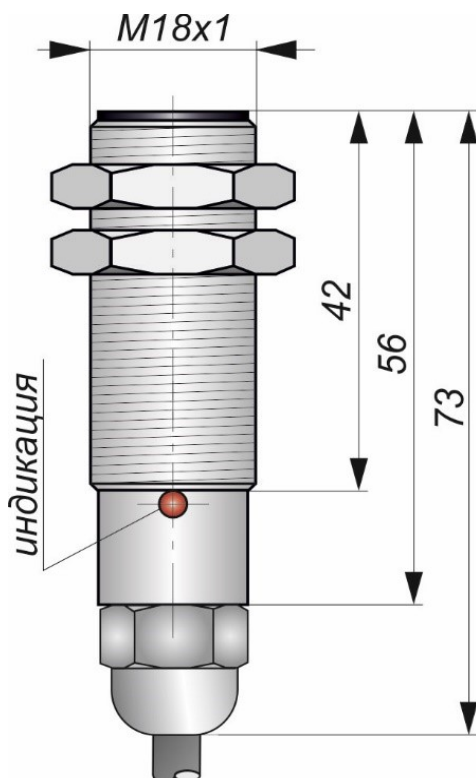
Габаритный чертеж
