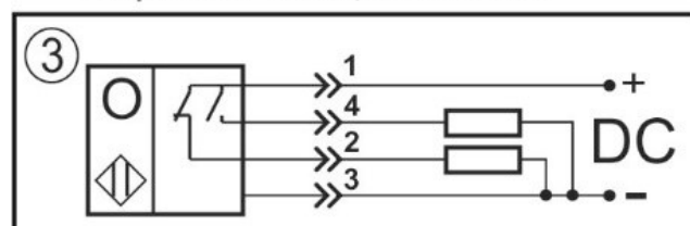
Переключающий контакт
