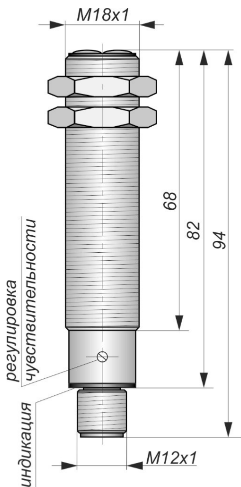
Габаритный чертеж
