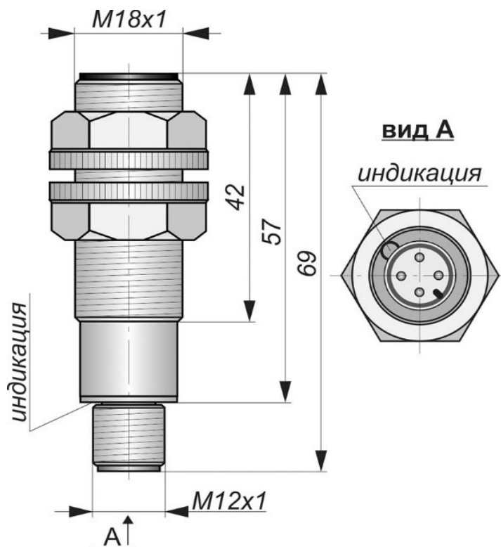
Габаритный чертеж
