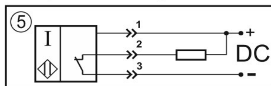
Цоколевка разъема
