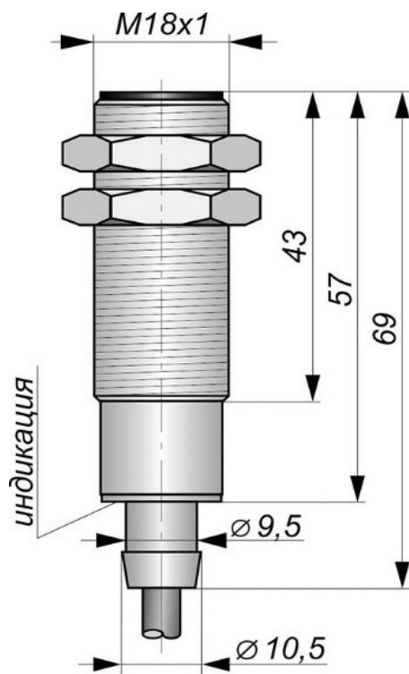
Габаритный чертеж
