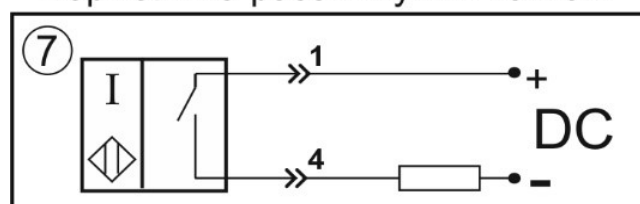
Нормально-разомкнутый контакт
