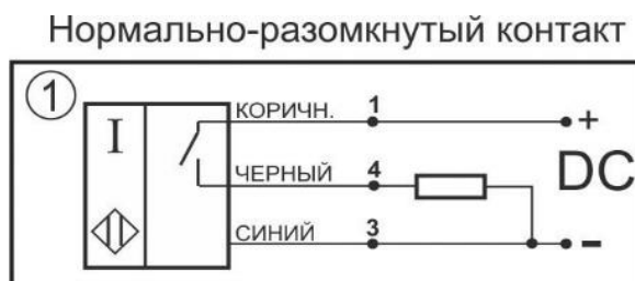
Схема соединения
