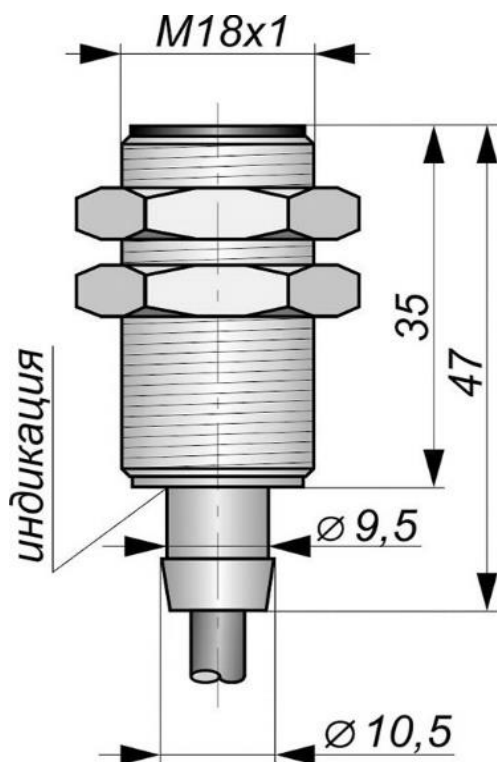
Габаритный чертеж
