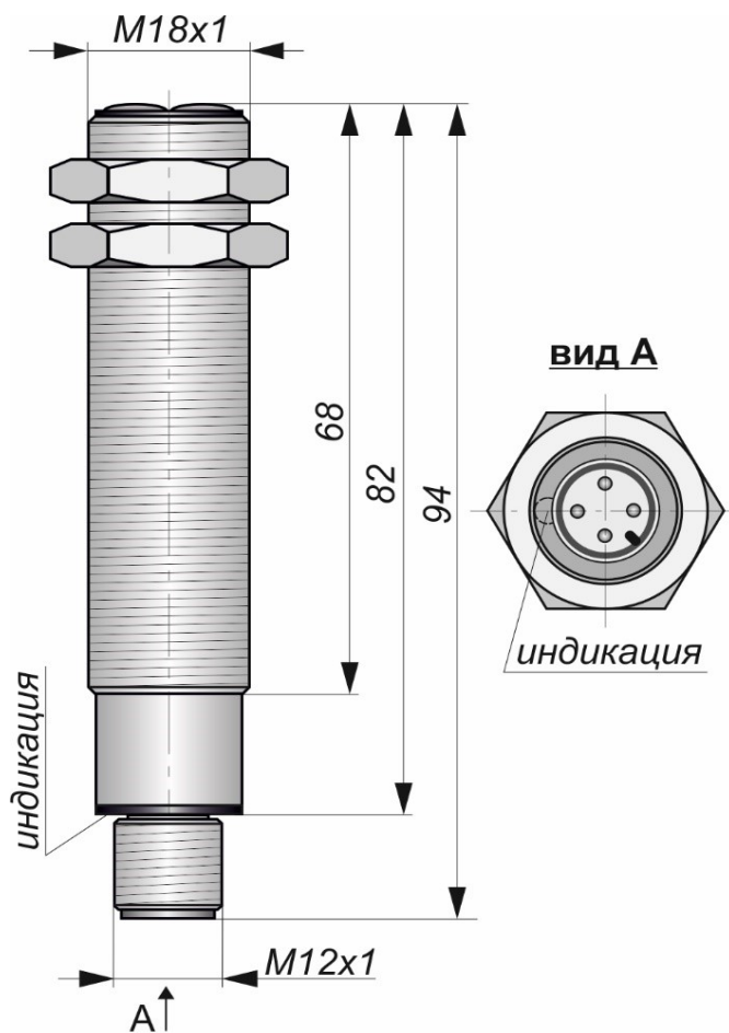
Габаритный чертеж
