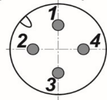
Цоколевка разъема
