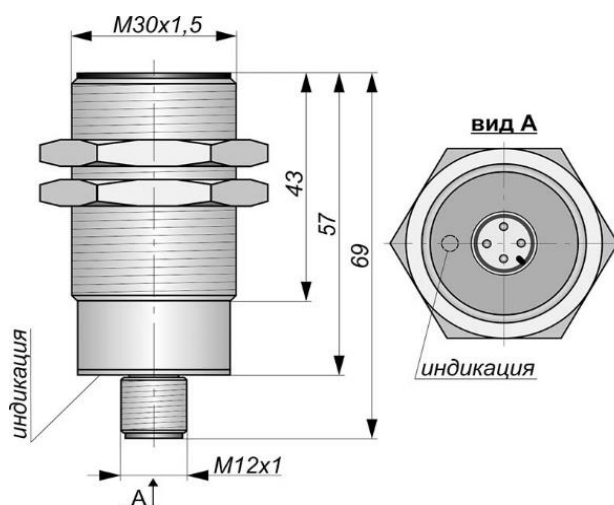
Габаритный чертеж
