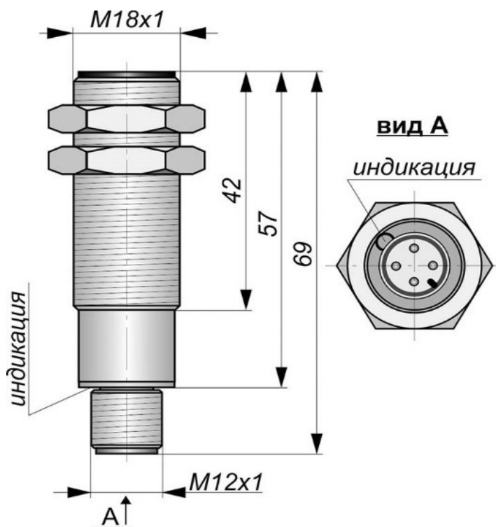
Габаритный чертеж
