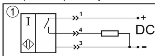
Цоколевка разъема
