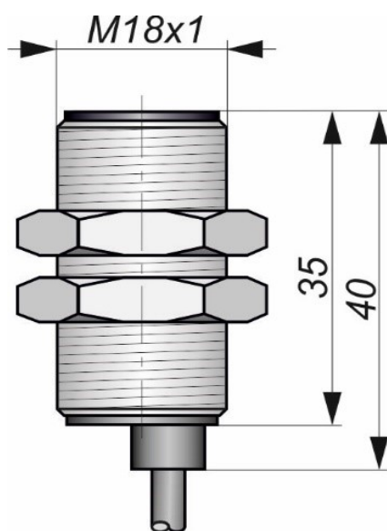
Габаритный чертеж
