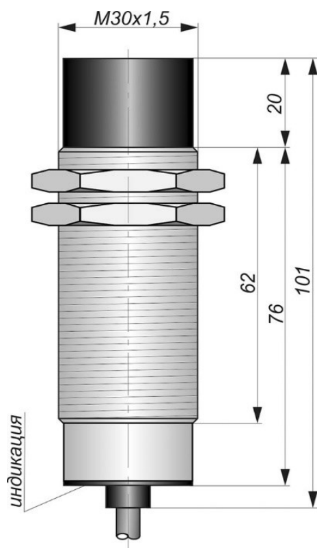
Габаритный чертеж
