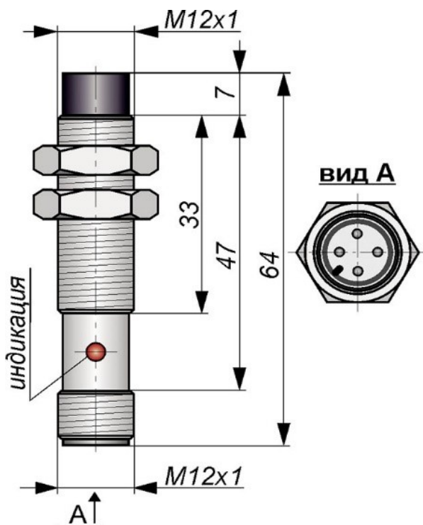
Габаритный чертеж
