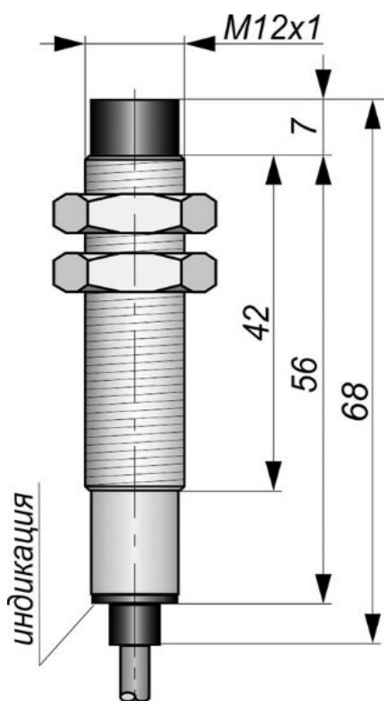
Габаритный чертеж
