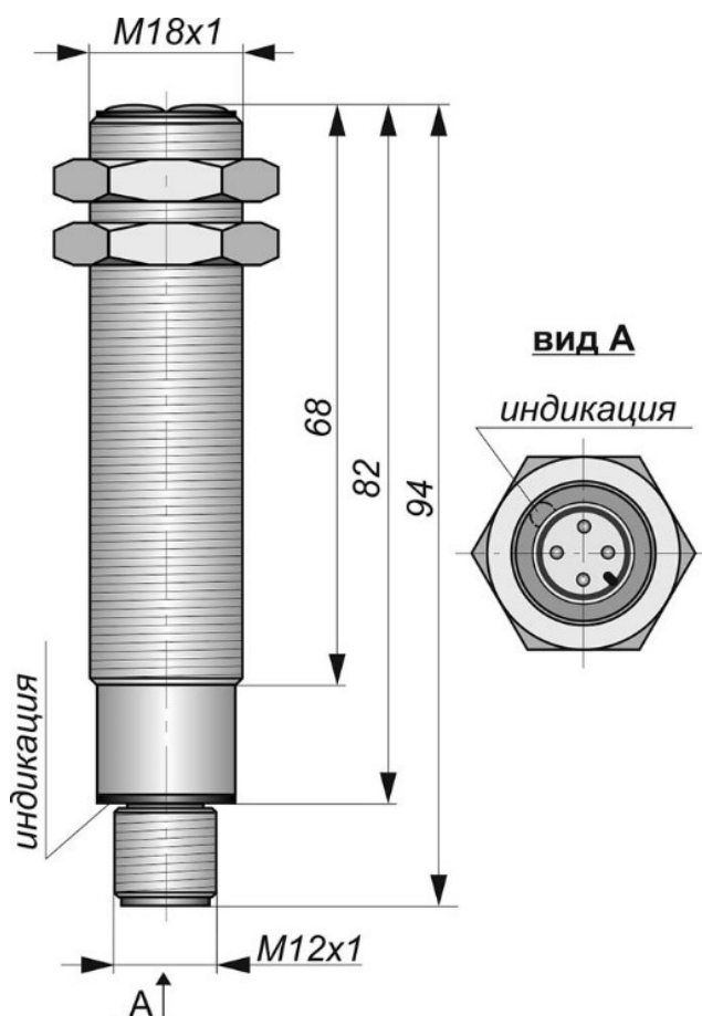
Габаритный чертеж
