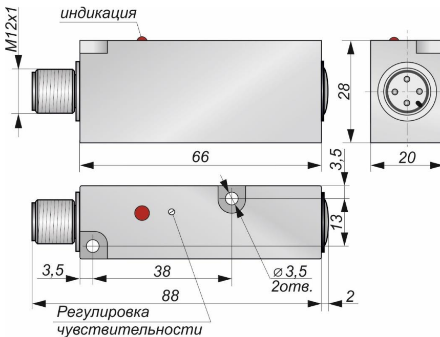
Габаритный чертеж
