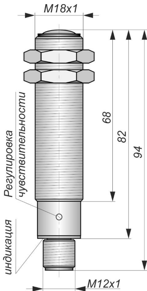
Габаритный чертеж
