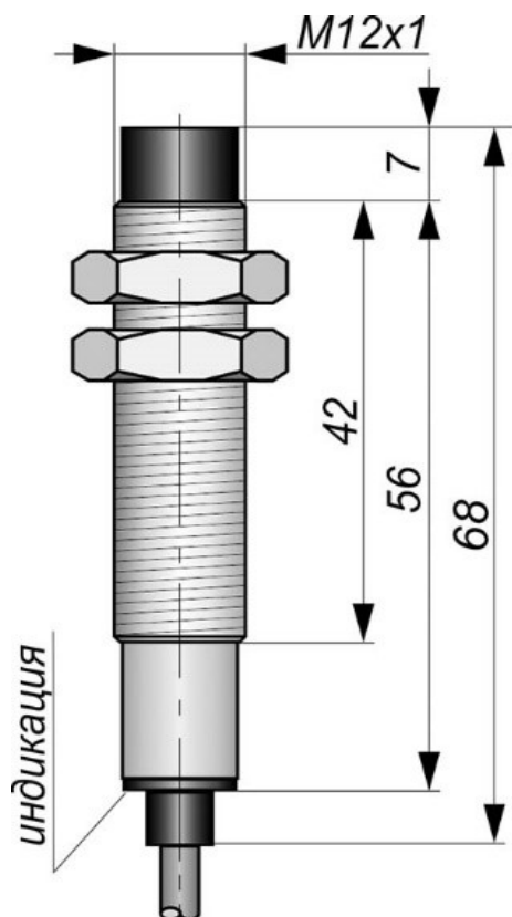
Габаритный чертеж
