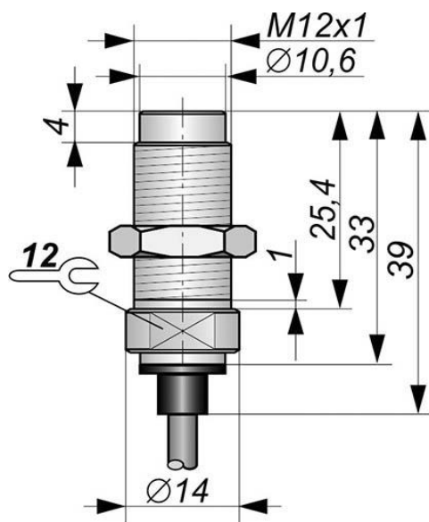
Габаритный чертеж
