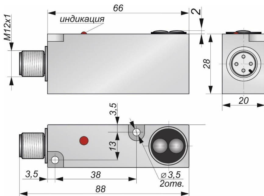
Габаритный чертеж
