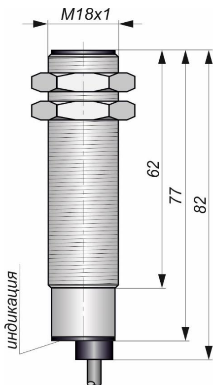
Габаритный чертеж
