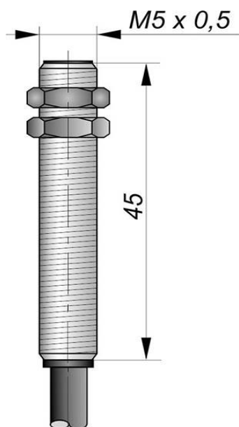
Габаритный чертеж
