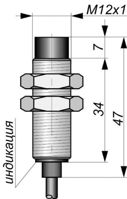
Габаритный чертеж
