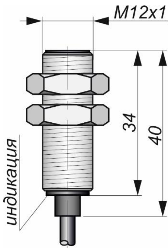
Габаритный чертеж
