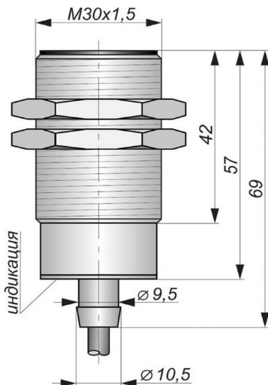
Габаритный чертеж
