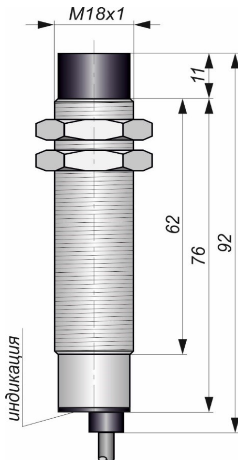
Габаритный чертеж
