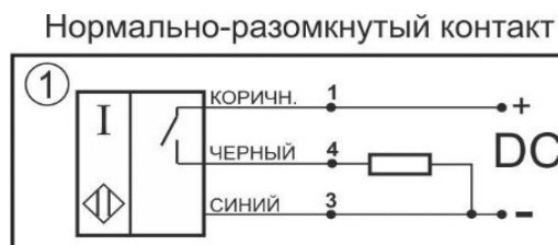
Схема соединения
