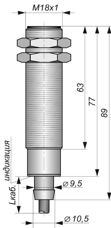
Габаритный чертеж
