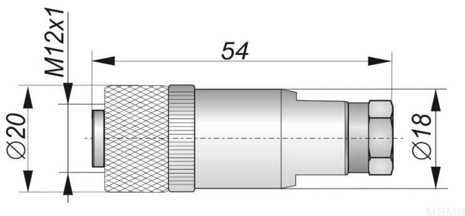
Габаритный чертеж
