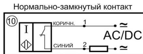
Схема соединения
