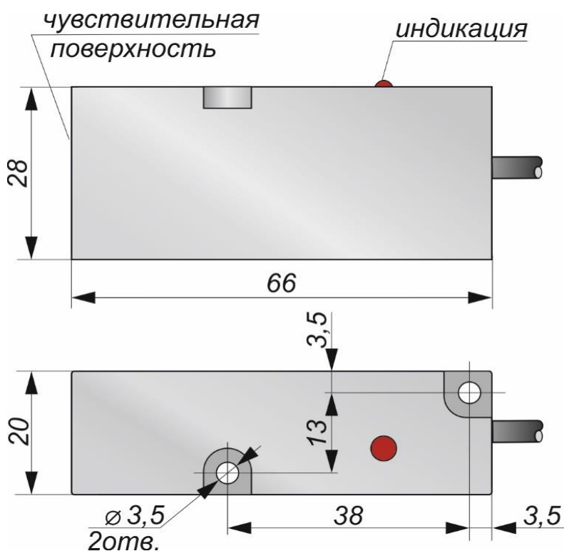
Габаритный чертеж
