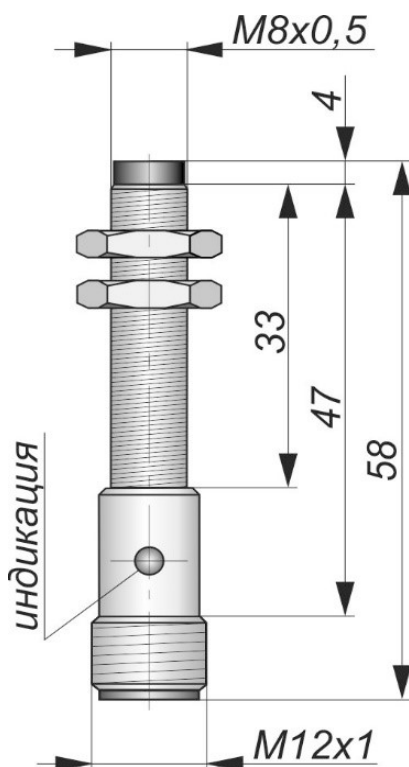
Габаритный чертеж
