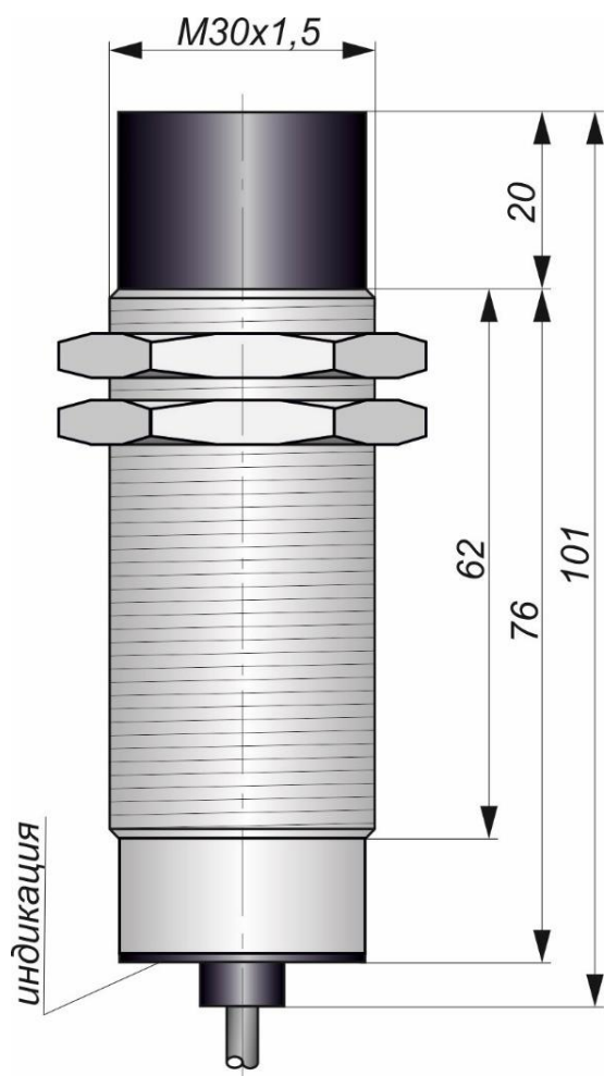
Габаритный чертеж
