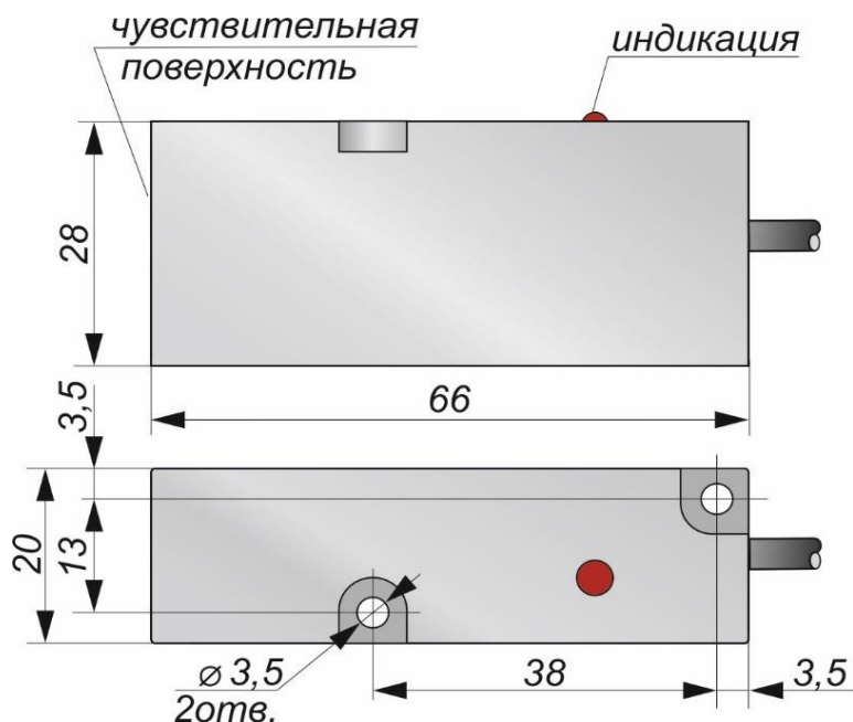
Габаритный чертеж
