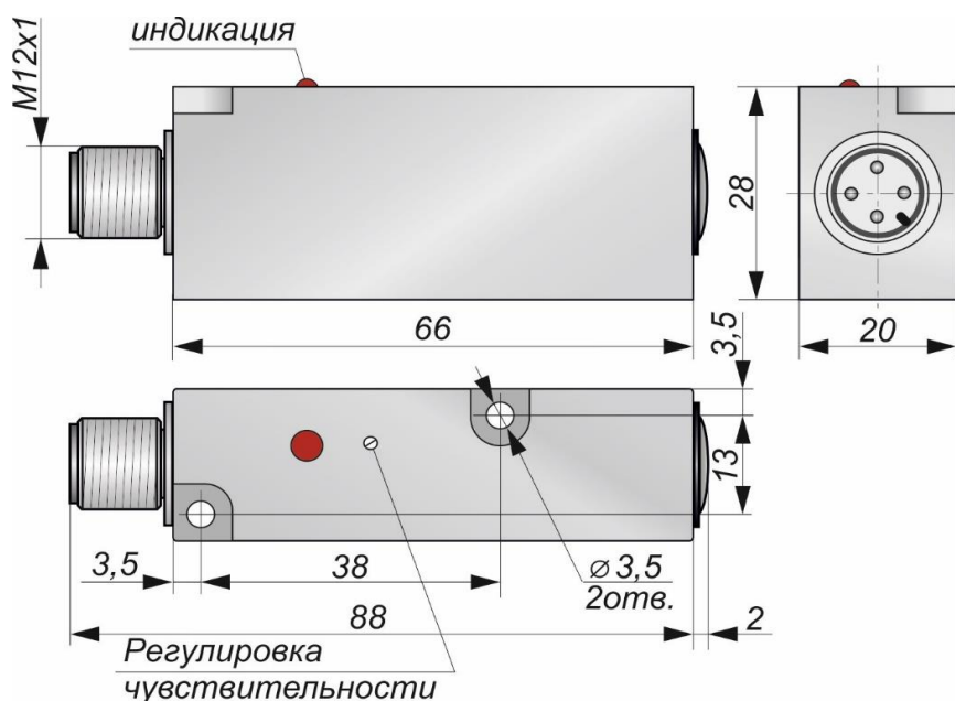
Габаритный чертеж
