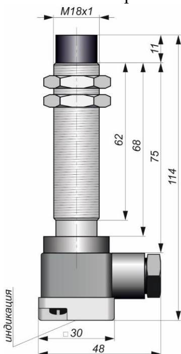
Габаритный чертеж
