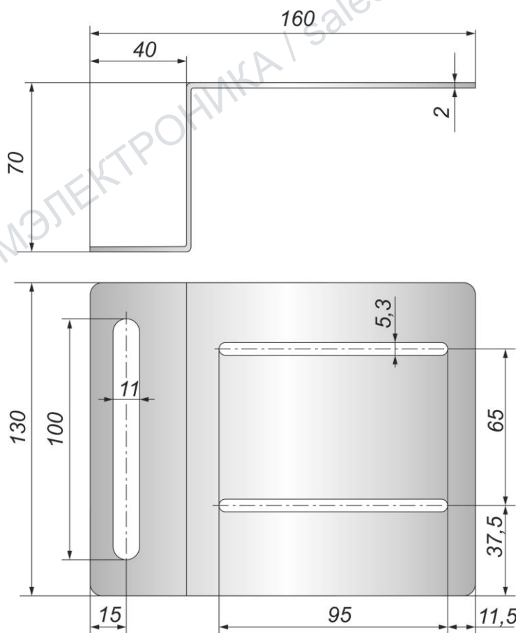
Габаритный чертеж
