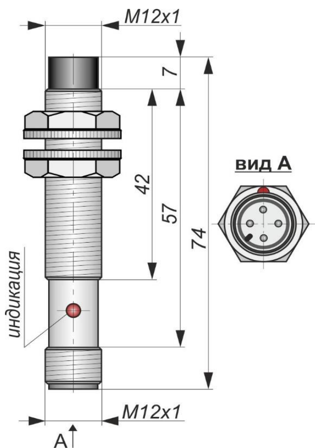
Габаритный чертеж
