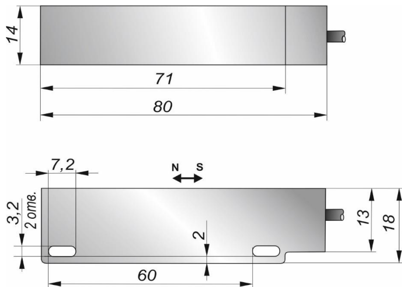
Габаритный чертеж
