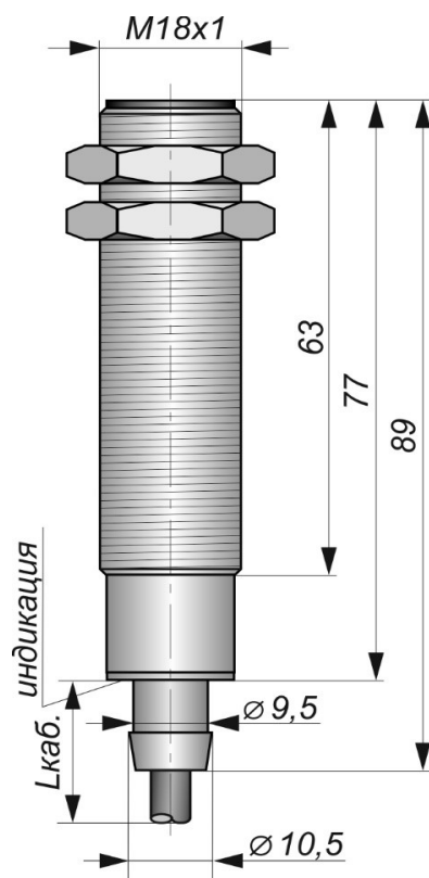
Габаритный чертеж
