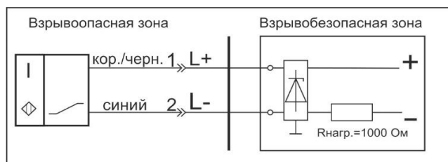
Цоколевка клеммной колодки
