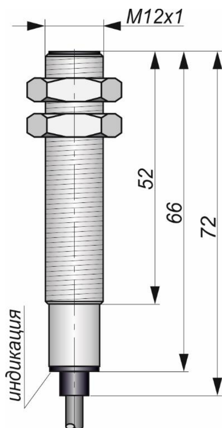
Габаритный чертеж
