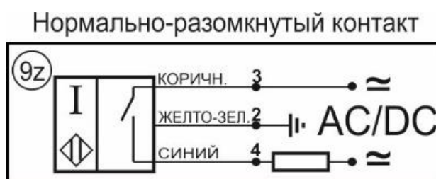
Схема соединения
