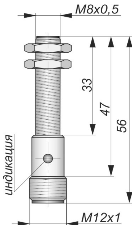
Габаритный чертеж
