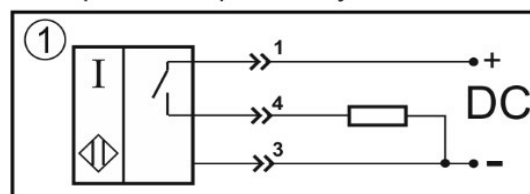
Цоколевка разъема
