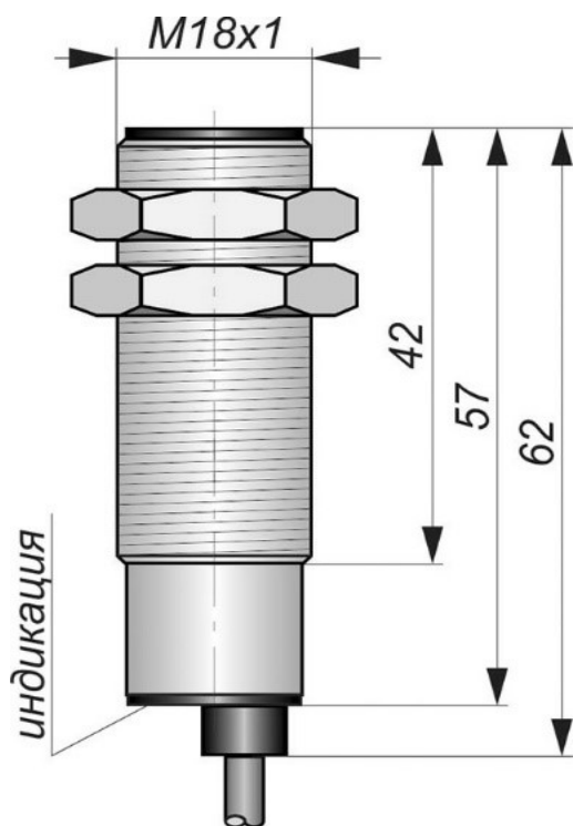
Габаритный чертеж
